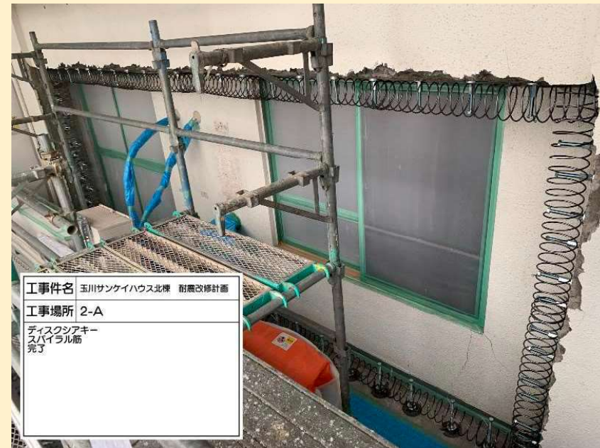
②工事中 (アンカー工事 完了状況)
